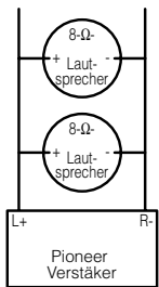
4-Ω-Überbrückungsmodus
